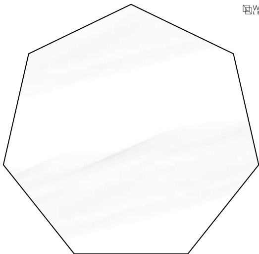
Liczba podzielna przez 7
