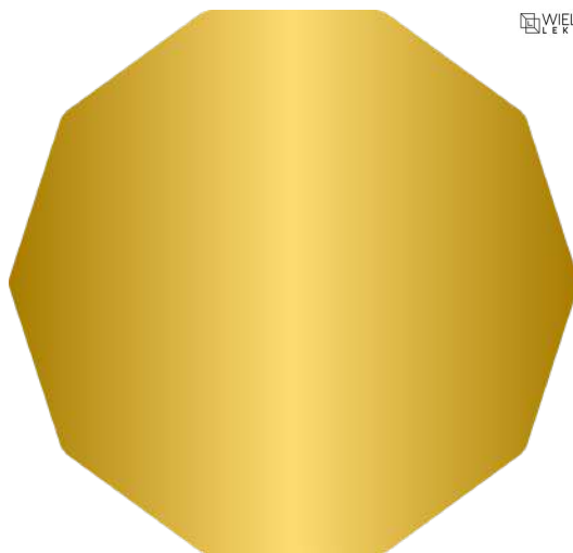
Liczba podzielna przez 10
