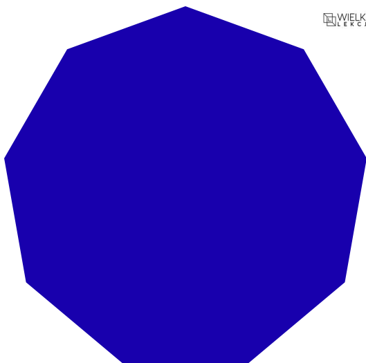
Liczba podzielna przez 9
